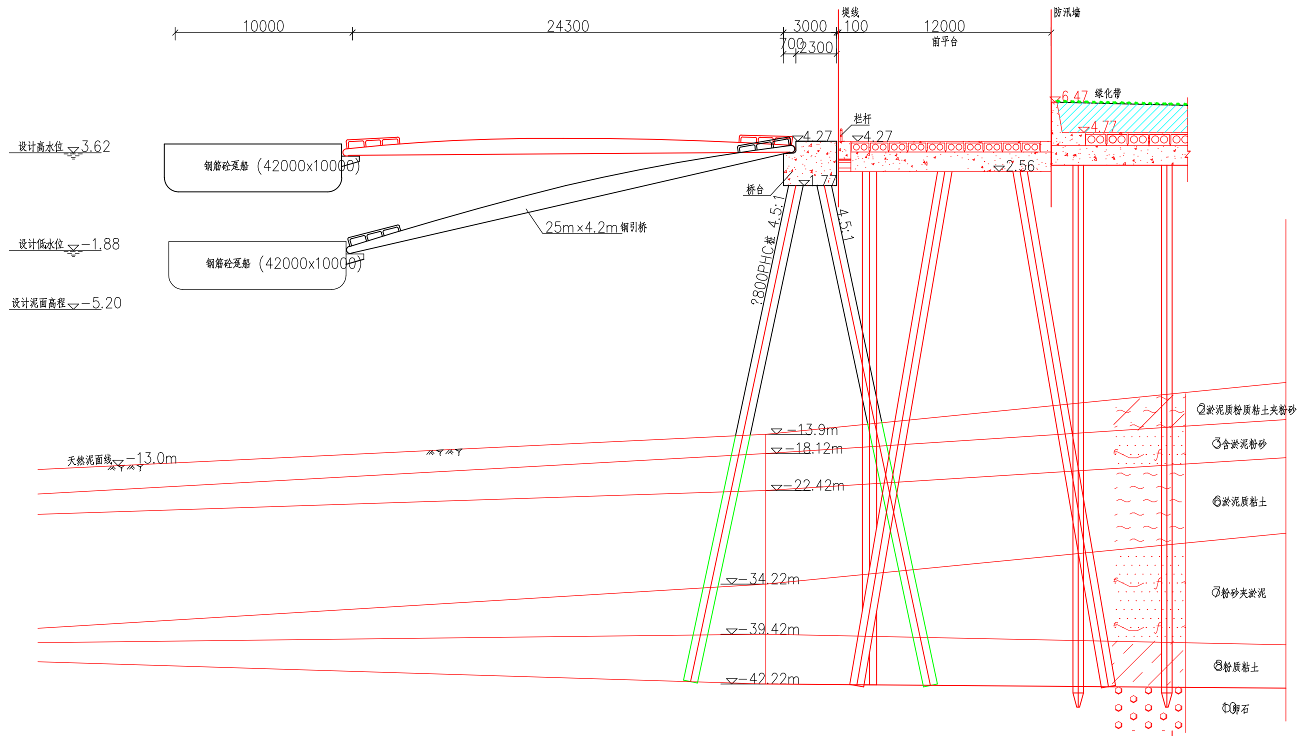
浮码头断面图
